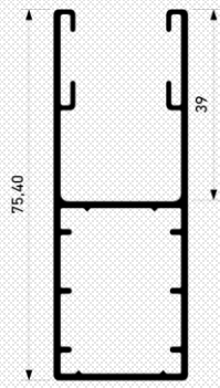
MONOBLOC 250 / 300
