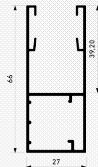
MONOBLOC 150 / 180 / 205
