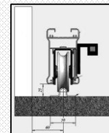
GALETS AVEC RENFORTS DE FIXATION POUR CREMAILLIERE
