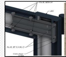
STRUCTURE RENFORCÉE
